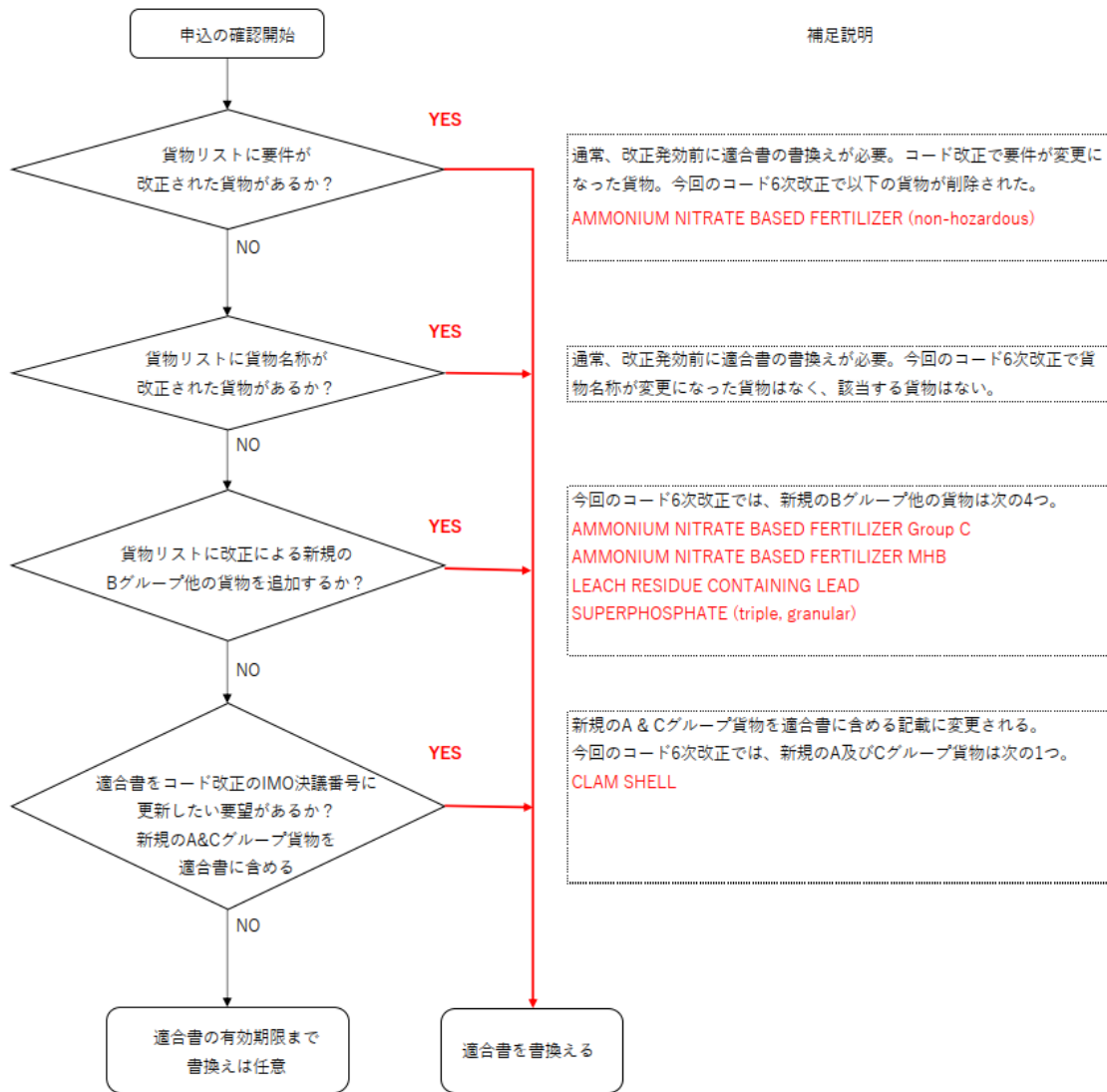
図1. IMSBC Code適合書の書換え要否のフローチャート
