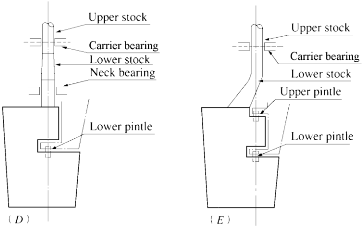
Fig. 4.2.1.1-1 Mariner-type Rudders
