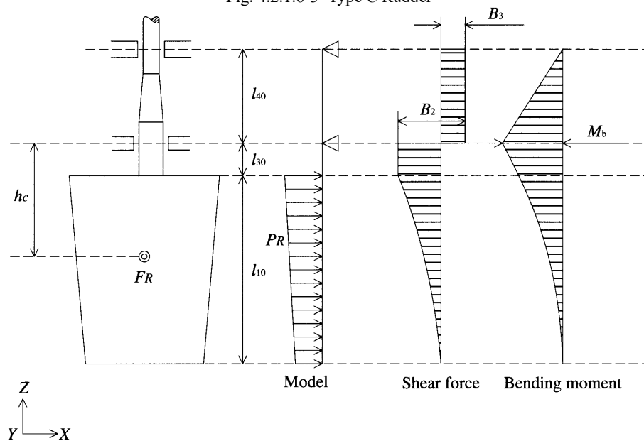
Fig. 4.2.1.6-3 Type C Rudder
