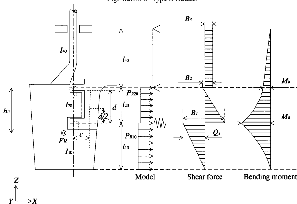
Fig. 4.2.1.6-5 Type E Rudder
