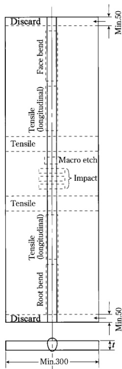
(D) Test Assembly for KL9N53 or KL9N60
