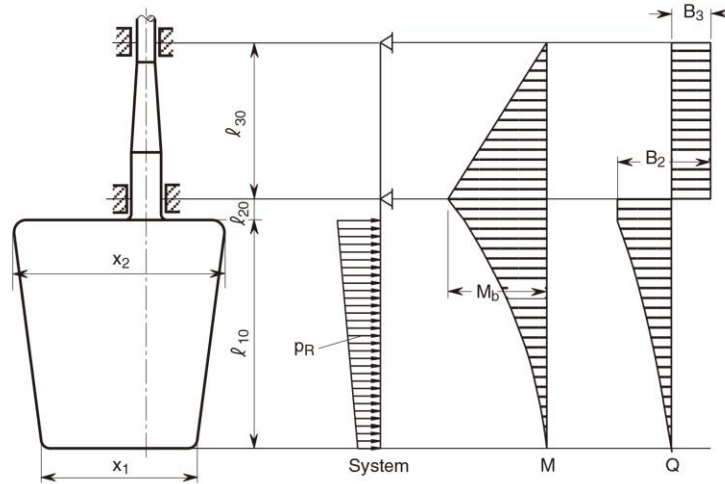
Fig. 6 Spade Rudder
