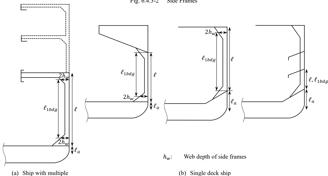
Fig. 6.4.3-2 Side Frames
