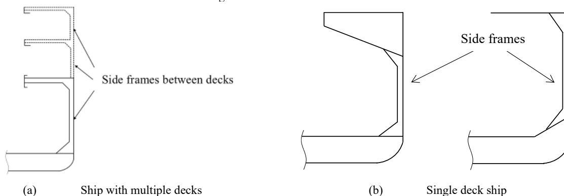
Fig. 6.4.3-1 Side Frames
