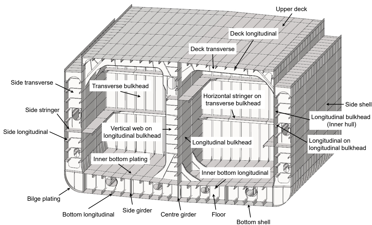
Fig. 1.4.5-8 Tanker
