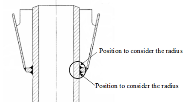
Fig. 11.5.1-5 Fillet Radius of Fillet Weld
