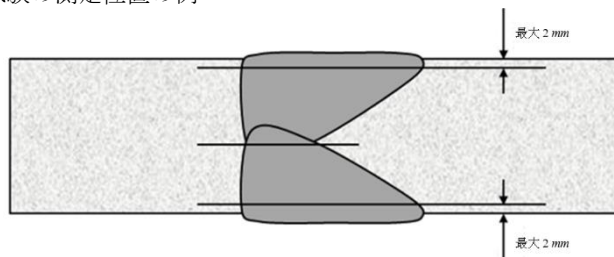
(2) 開先形状が K 形
