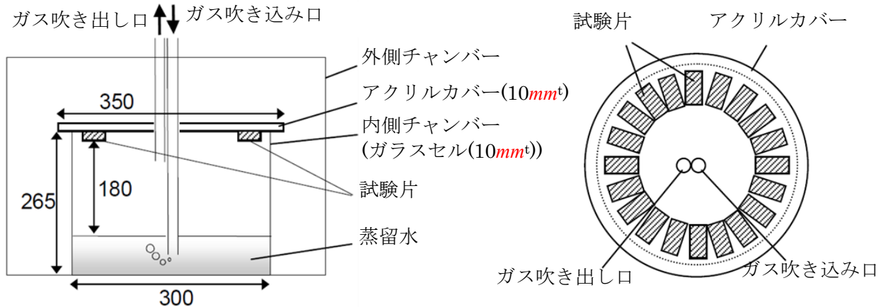
図 1.1-2. 上甲板用模擬腐食試験装置の例
