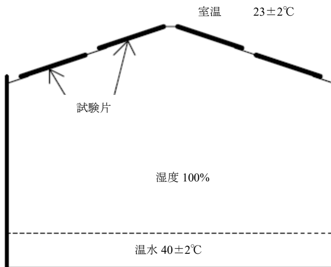
図 4.2-2. 結露装置
