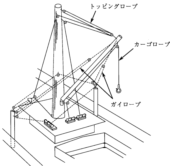
1 トッピング式デリッククレーン装置
