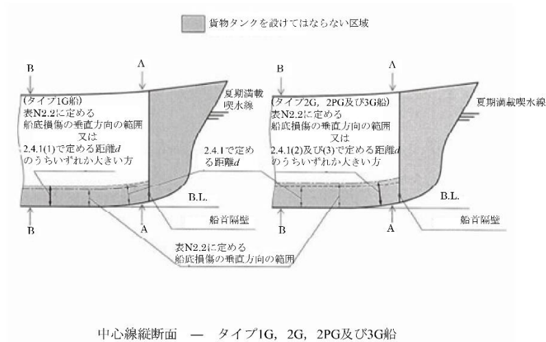
図 N2.1 貨物タンクの配置要件
