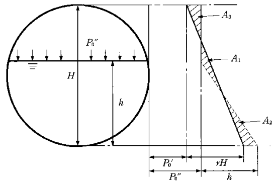
図 N4.21.5-3. 圧力荷役状態の内圧分布の模擬
