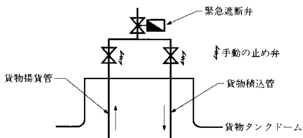
図 N5.5.2 止め弁と緊急遮断弁の併設
