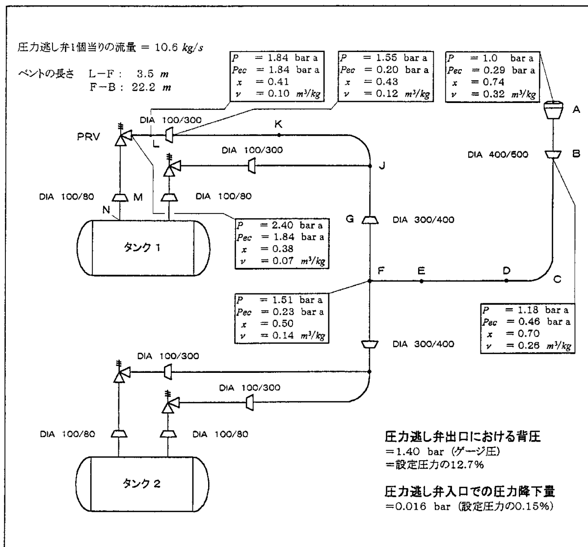
図 2 二相流における圧力逃し弁に対する規定容量での各節における各状態量（プロパンの場合）
