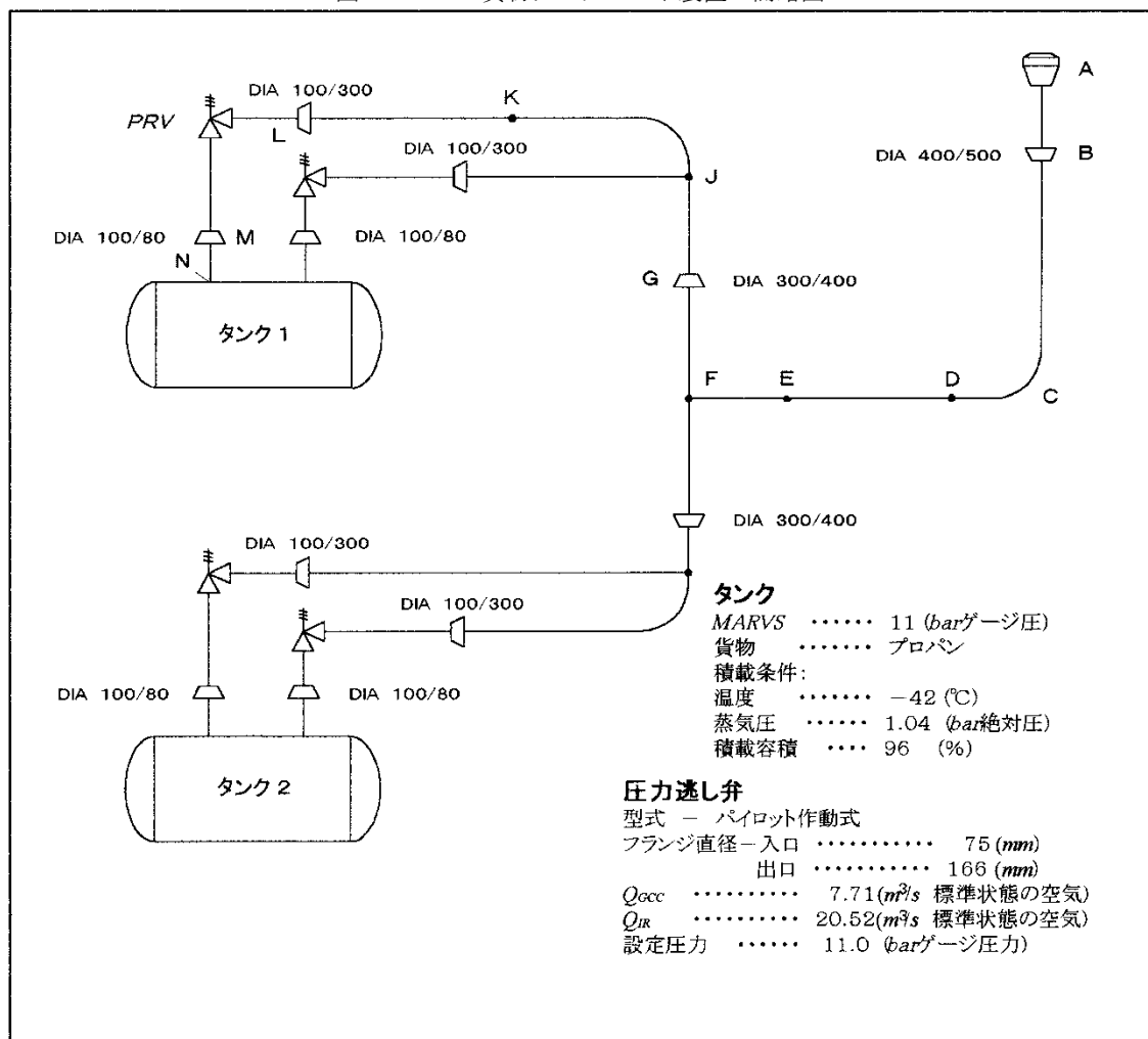
図 1 貨物タンクベント装置の簡略図
