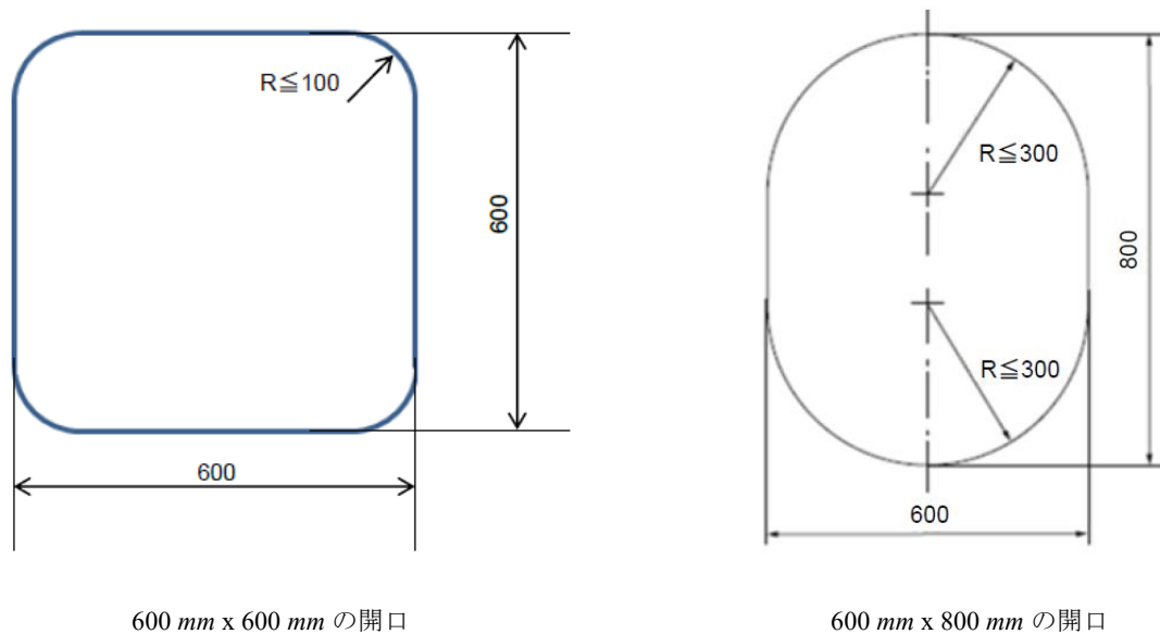
図 N3.5.3-2. 垂直面に設ける交通口の例
