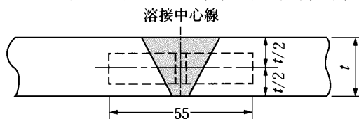
図 M6.4 衝撃試験片の採取位置 ( t : 板厚, 単位 mm)
