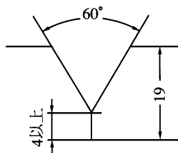
(イ) 多層盛突合せ
