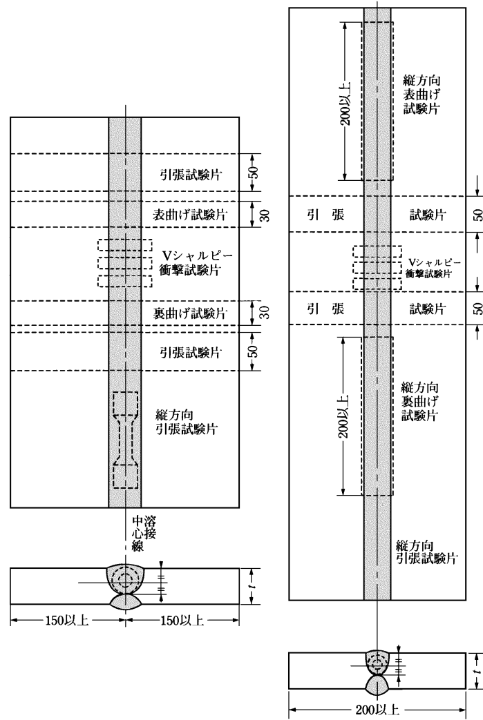
図 M6.9 二層盛溶接法の突合せ溶接試験材 ( t : 板厚, 単位 mm )
