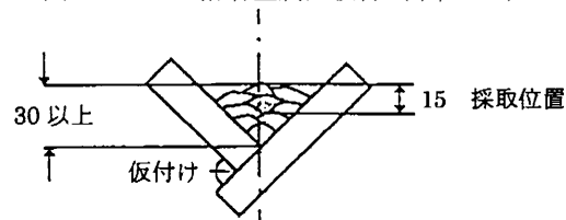
図 M6.19 溶着金属試験材 (単位 mm)
