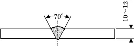
片面溶接の場合
