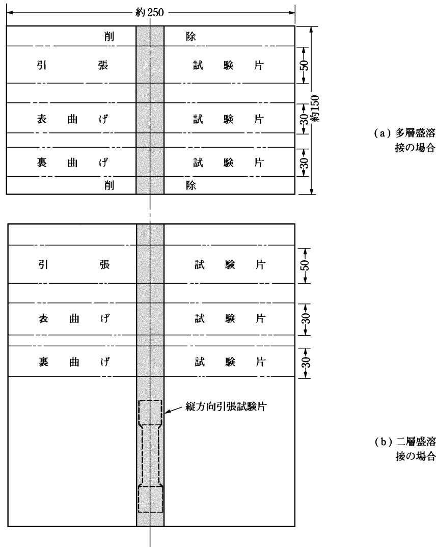
図 M6.18 サブマージアーク自動溶接材料の突合せ溶接試験材 (単位 mm)
