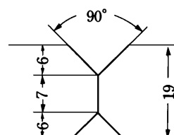
(ハ) 二層盛突合せ, 板厚=19
