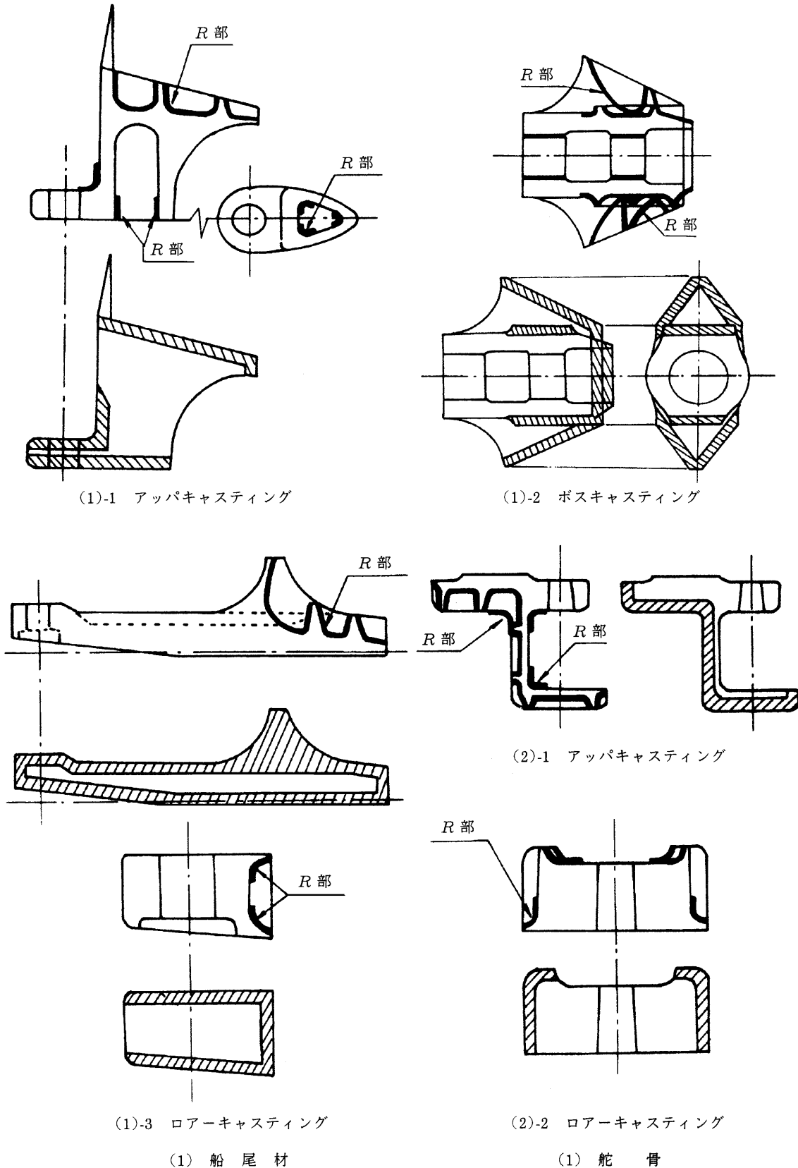
図3 磁粉探傷検査の適用例
