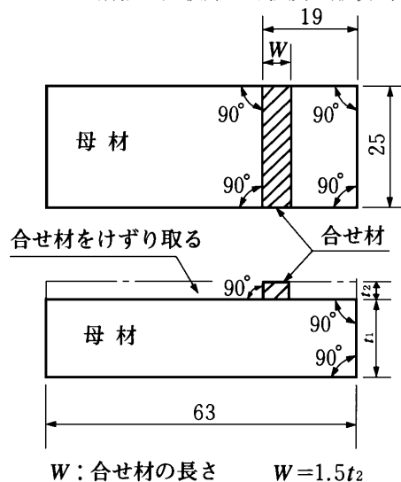
図 K3.3 せん断強さ試験片の寸法及び形状 (単位 mm)
