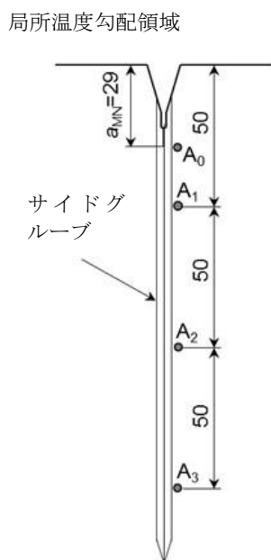
図 5 局所温度勾配領域及び熱電対 A_0 の位置
