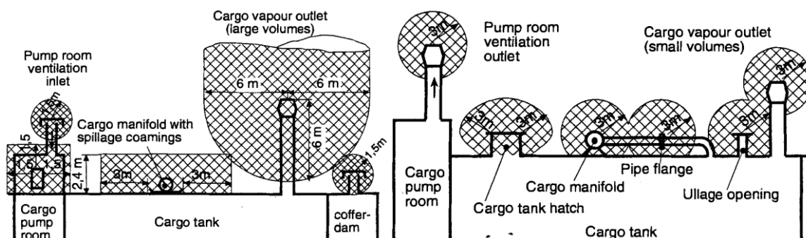
図 H4.3.1(3) 2 種危険場所の例
