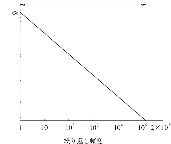
図 GF6.3 簡易化した荷重分布 ～15日
