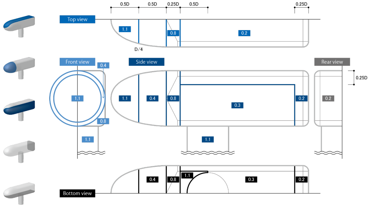
図 D.2 等価風圧係数【風向：-15°～+15°・正值】
