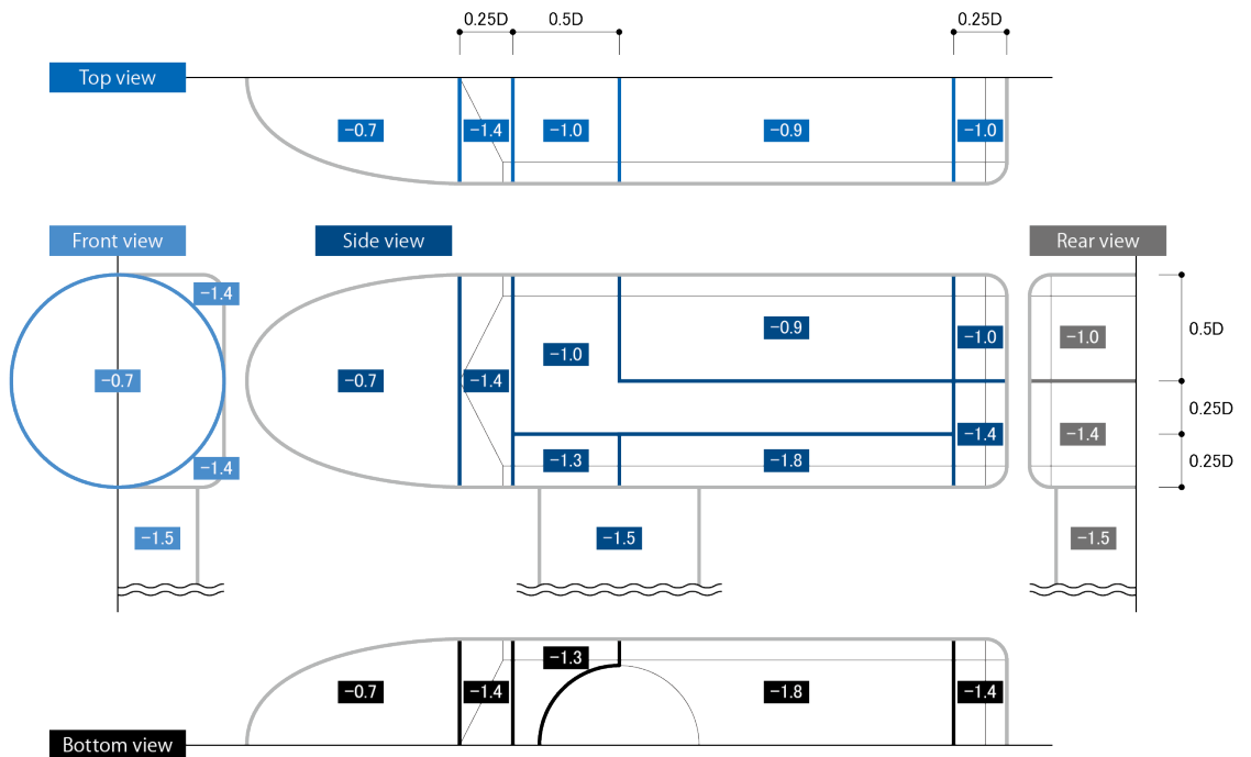
図 D.3 等価風圧係数【風向：-15°～+15°・負値】
