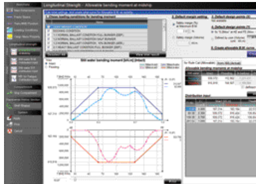
CSR (規範) 用的介面
