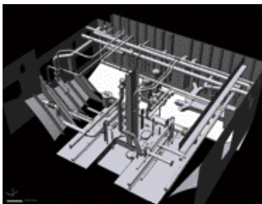
點群資料產生的3D模型
