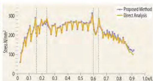
总应力（中拱） 13,000 TEU 的抗扭应力试验结果 集装箱船（修改后的指南）
