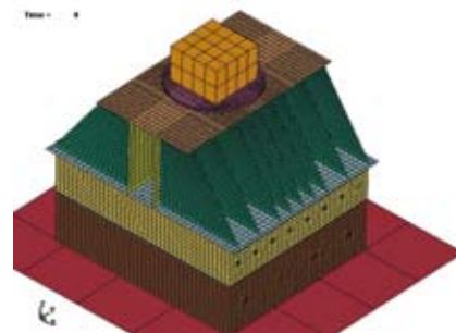
薄膜型LNG船储罐隔热构造上晃动载荷的计算机模拟测试
