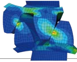
伞齿轮轮齿反复咬合的负荷测试
