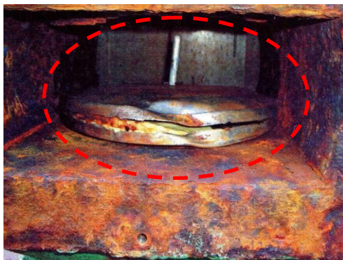
ディスクフロートの破損
