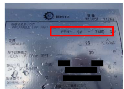
ダビット進水式の救命いかだの銘板
